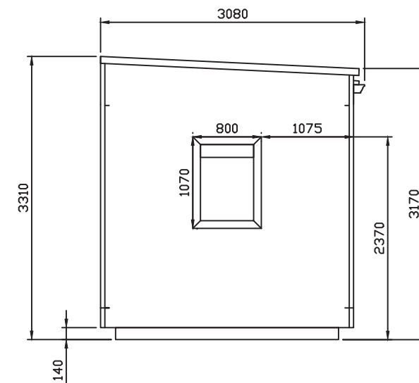
PIGNON DROIT
