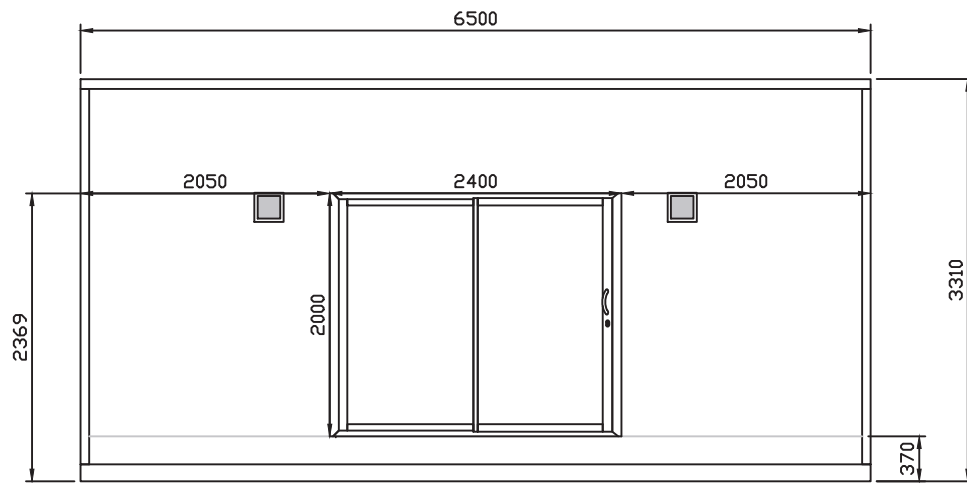
FAÇADE AVANT
