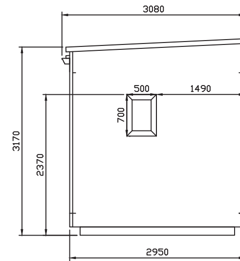
PIGNON GAUCHE
