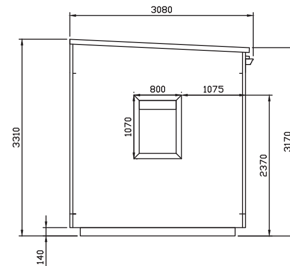
PIGNON DROIT
