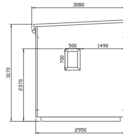
PIGNON GAUCHE
